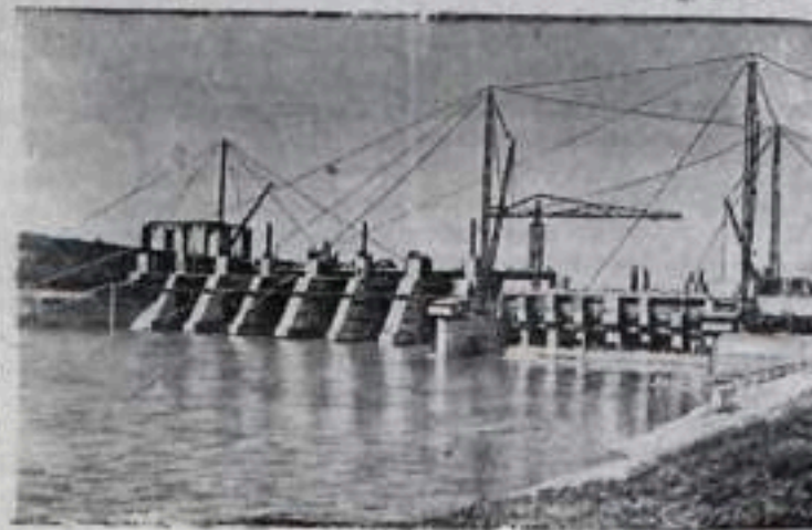
Молдавская ССР. На строительстве Дубоссарской ГЭС закончено сооружение плотины и начата одна из наиболее ответственных этапов работы—затопление котлована.
