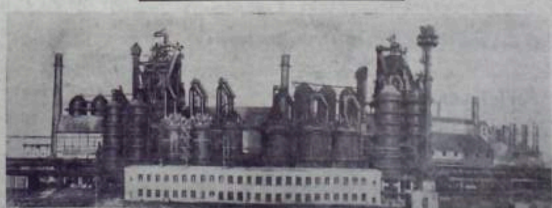
Вологодская область. Продолжается ввод в действие новых мощностей Череповецкого металлургического завода. Строители и монтажники готовят к сдаче в эксплуатацию новую доменную печь, оборудованную по последнему слову техники. НА СНИМКЕ: общий вид доменного цеха. Справа — действующая печь №1. Рядом новая печь №2.
