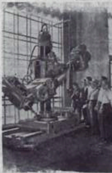
НА СНИМКЕ: в цехе «Станкостроение». Посетители осматривают переносный радиально-сверлильный станок модель 2П56, изготовленный на Одесском заводе радиальных станков. Наибольший диаметр сверления в стали равен 50 миллиметрам. Скорость шпинделя может изменяться от 14 до 850 оборотов в минуту. Фото Э. Евзелихина. Фотохроника ТАСС.
