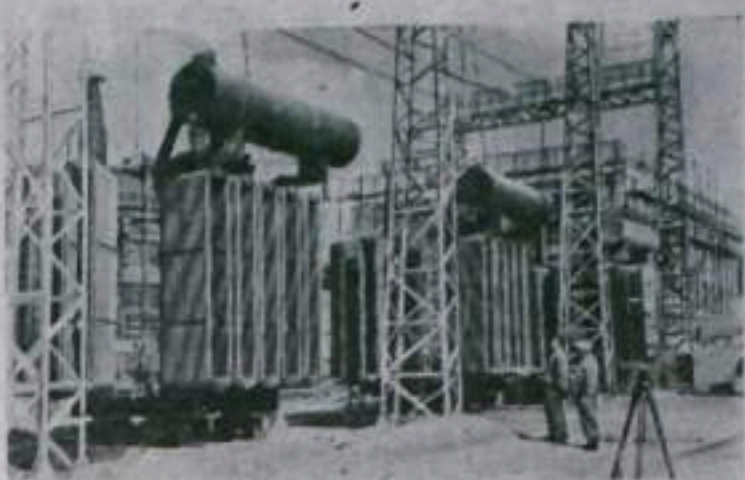
Московская область. В районе Ногинска заканчивается строительство подстанции, предназначенной для приема электроэнергии с Куйбышевской гидроэлектростанции. Первоначальное напряжение в 400.000 вольт будет понижаться до 220.000 и 110.000 вольт. Подстанция полностью оснащена отечественным оборудованием. НА СНИМКЕ: трансформаторная группа новой подстанции.
