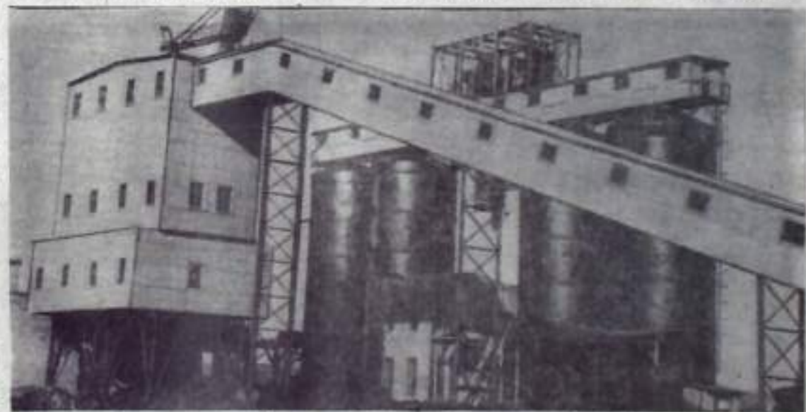
Строящийся автоматизированный бетоно-растворный завод.
