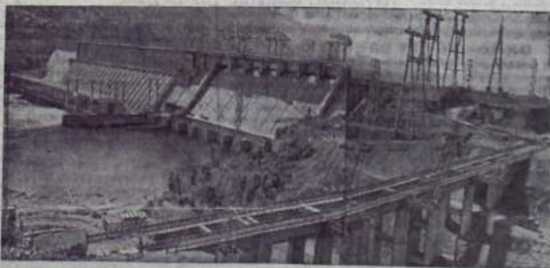
НА СНИМКЕ: Красноярская ГЭС со стороны строящегося судоподъемника. Фото Ю. БАРМИНА.
