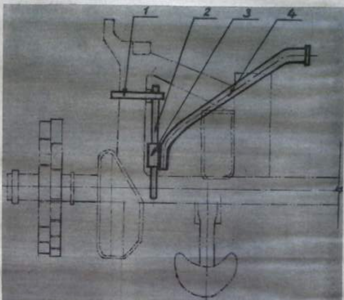
Измененное крепление тяговой штанги 1. Хомут 2. Стержень 3. Втулка 4. Штанга
