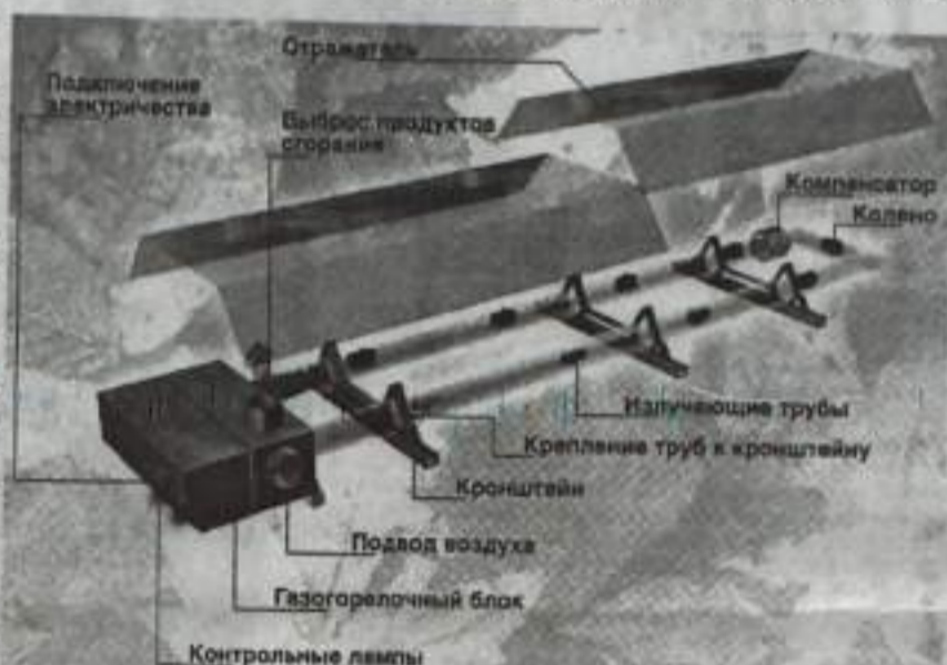
Устройство и принцип действия излучателя.
